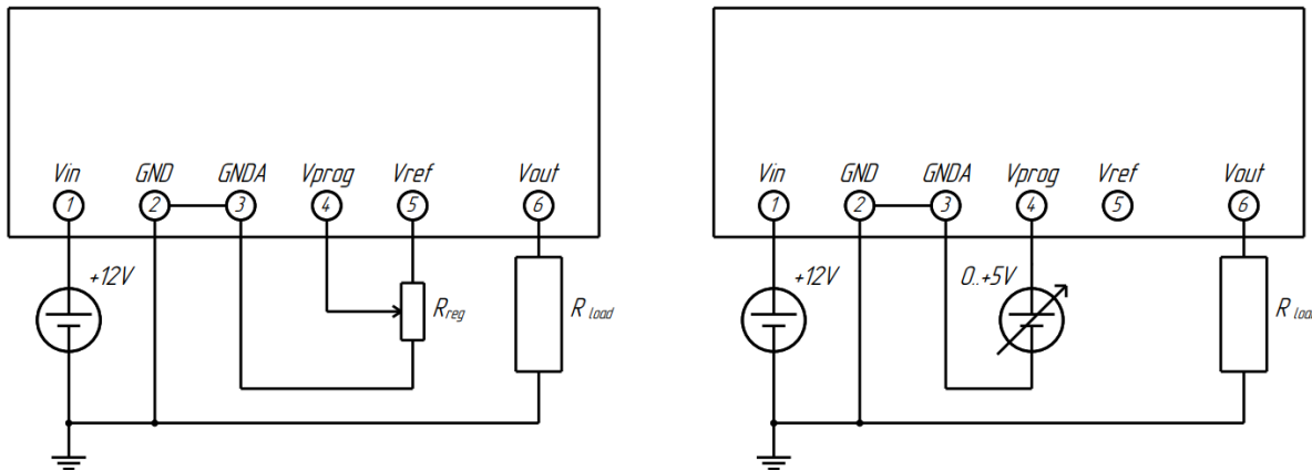
Рис.2 – Схема подключения
